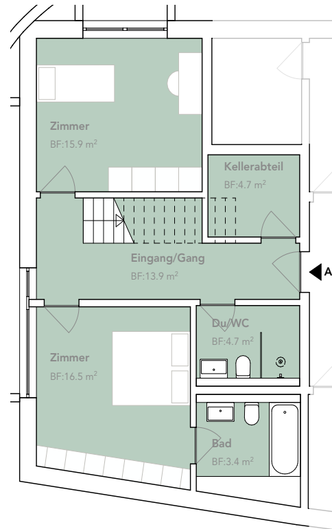
UNTERGESCHOSS
